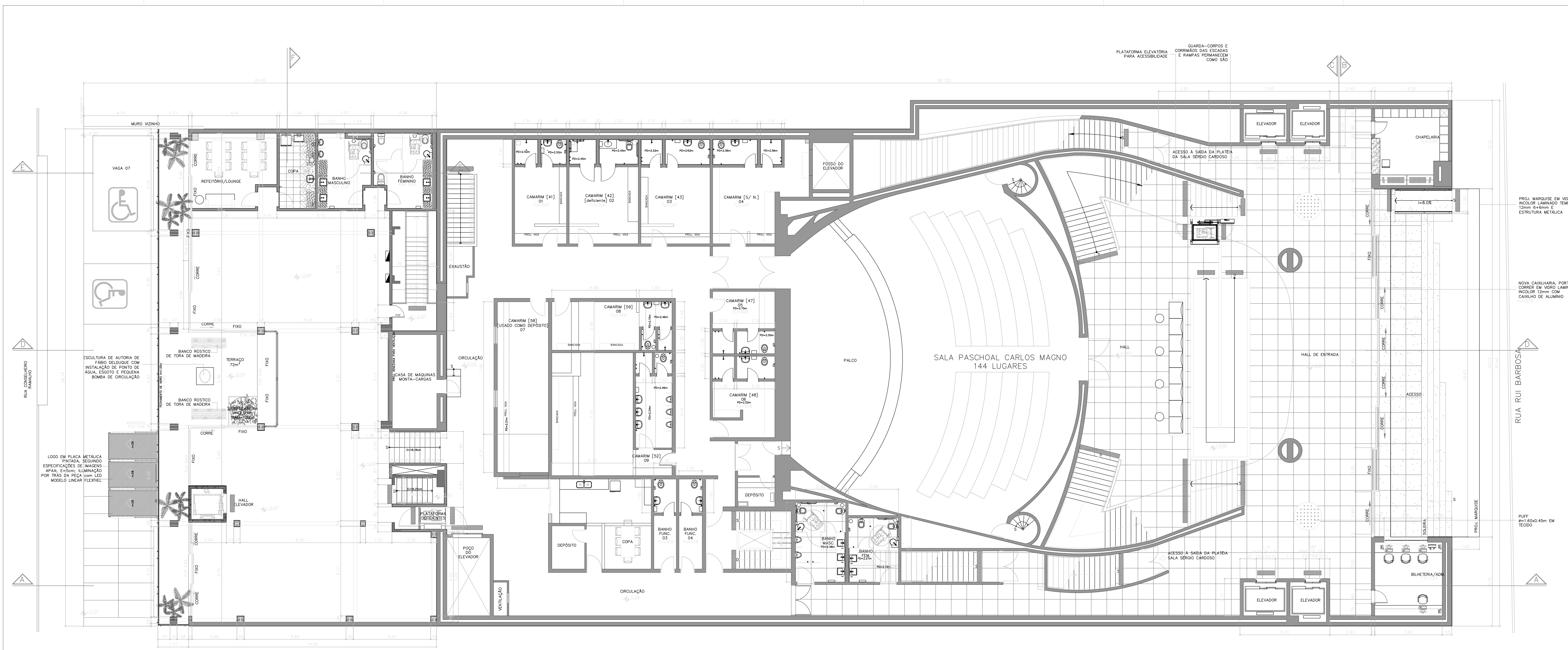
PLANTA 1ª PAV. – TERREO DA RUA RUI BARBOSA
