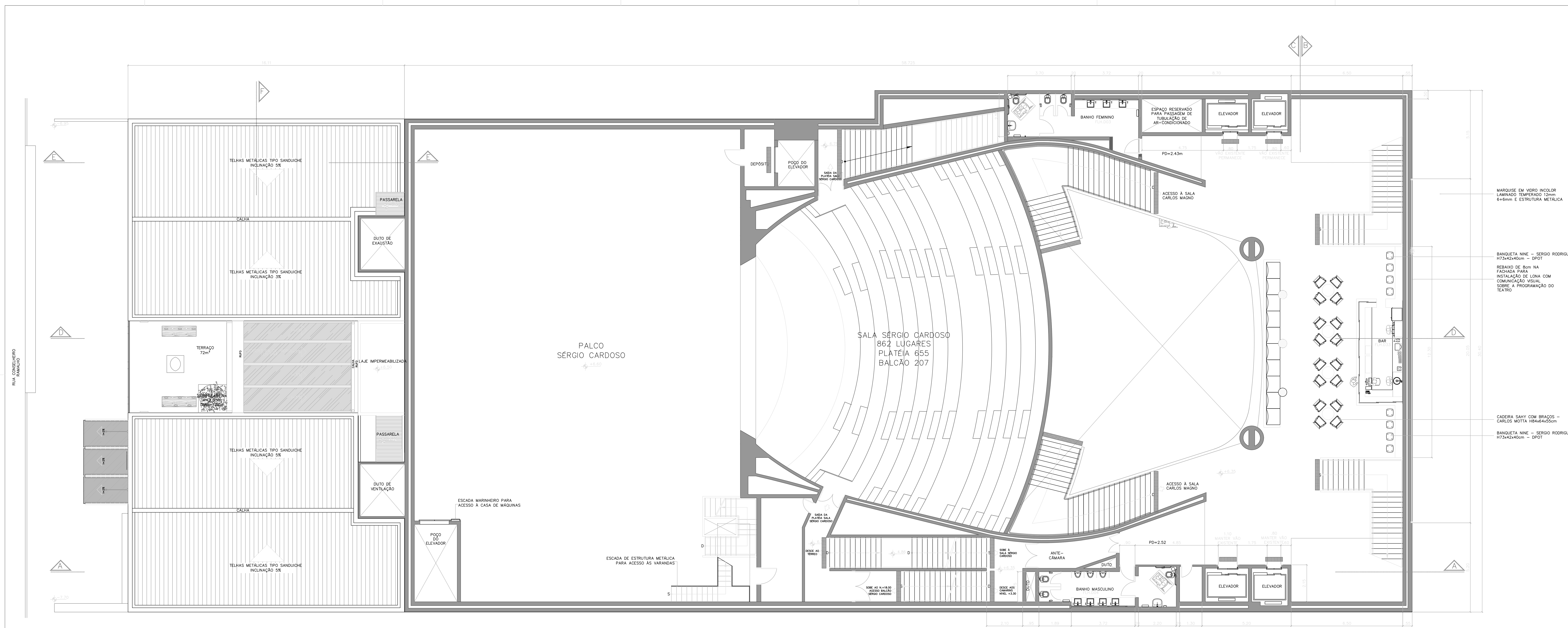
PLANTA 3ª PAV. – MEZANINO – NÍVEL +6.35 E PLANTA COBERTURA POSTERIOR
