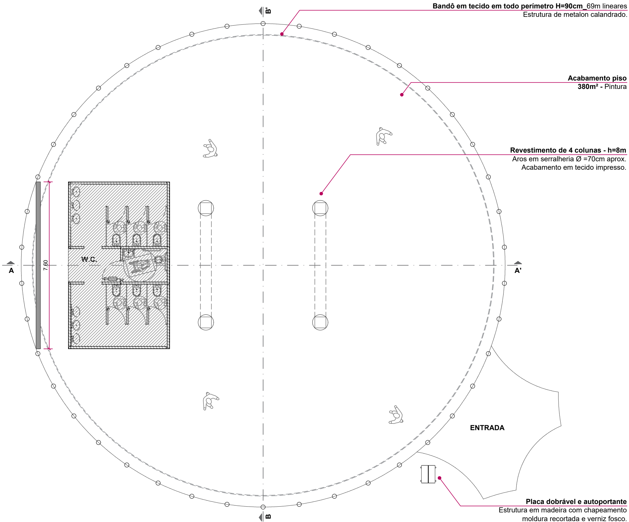
PLANTA TÉRREO
