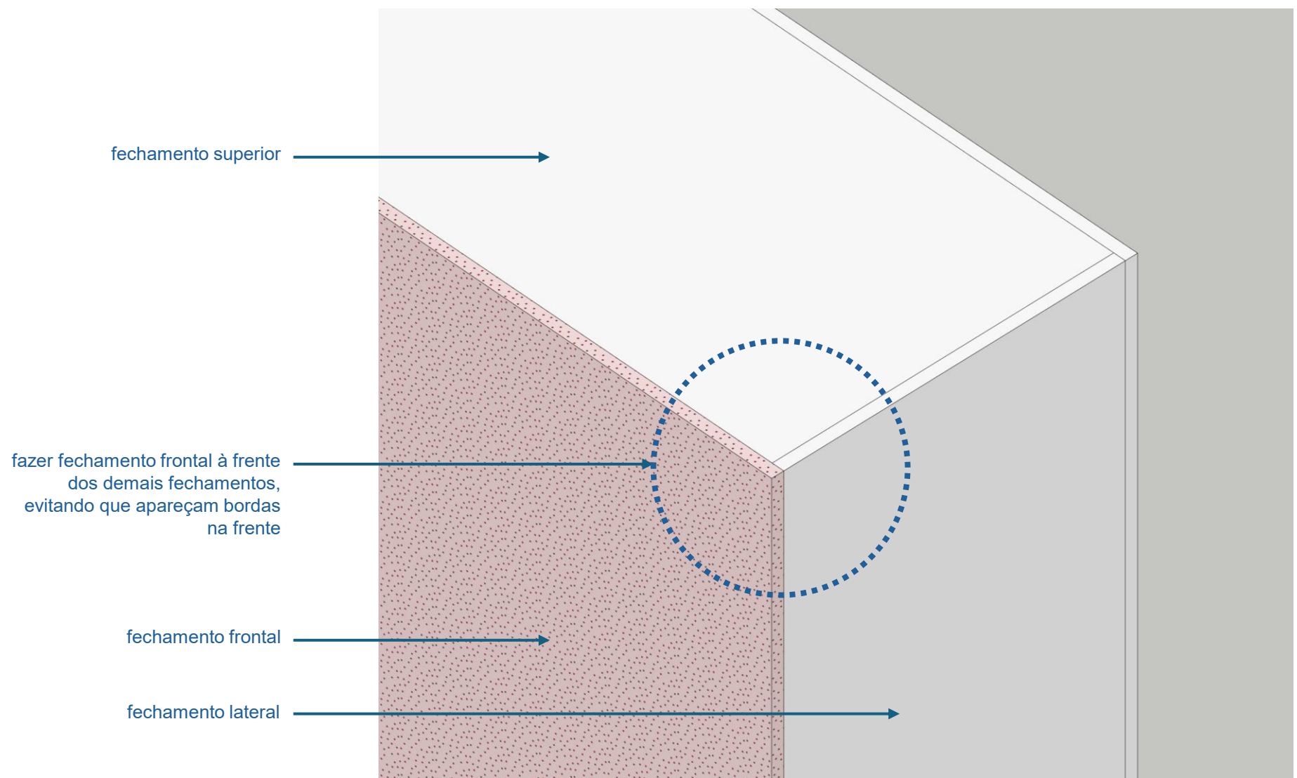
DETALHE DOS FECHAMENTOS DOS PAINÉIS DE FUNDO
