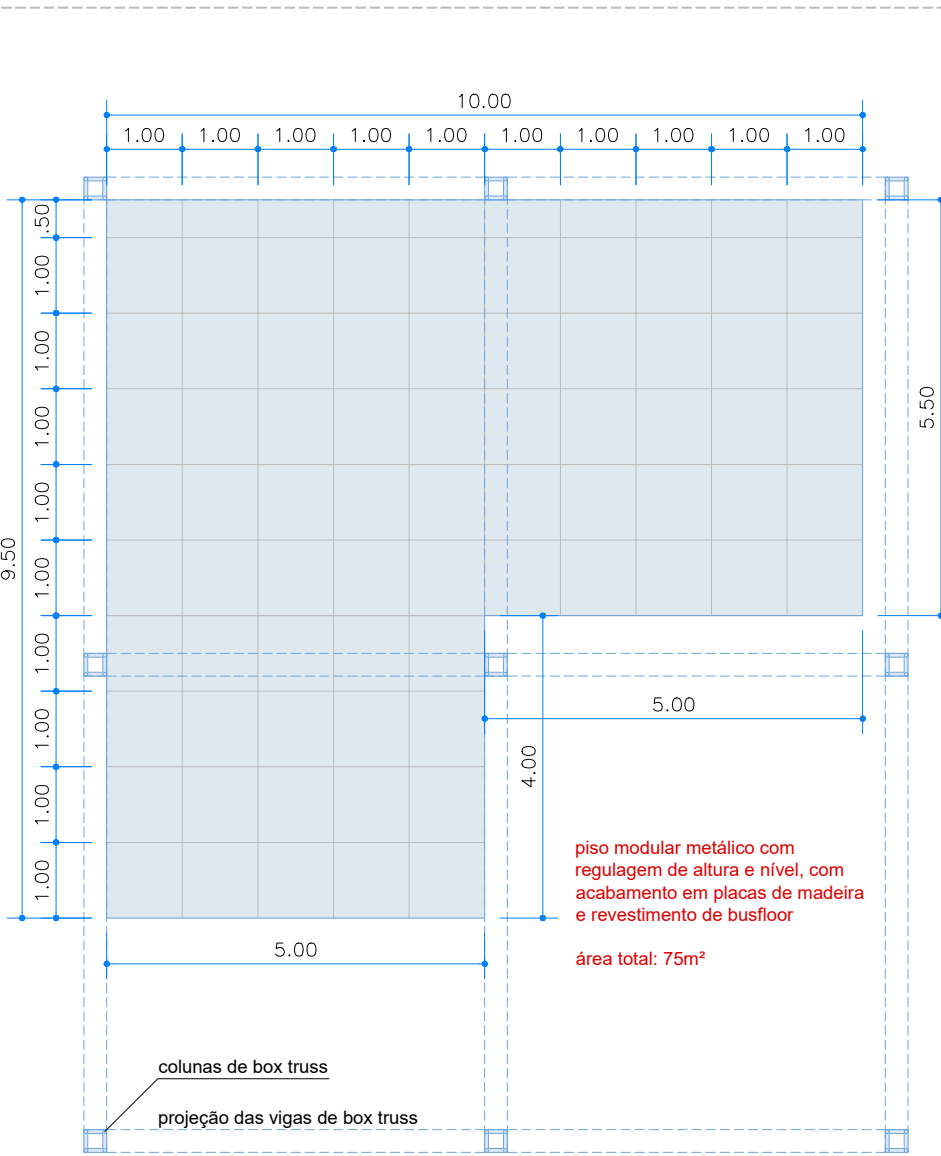
ampliação copa | planta de piso elevado escala 1:100
