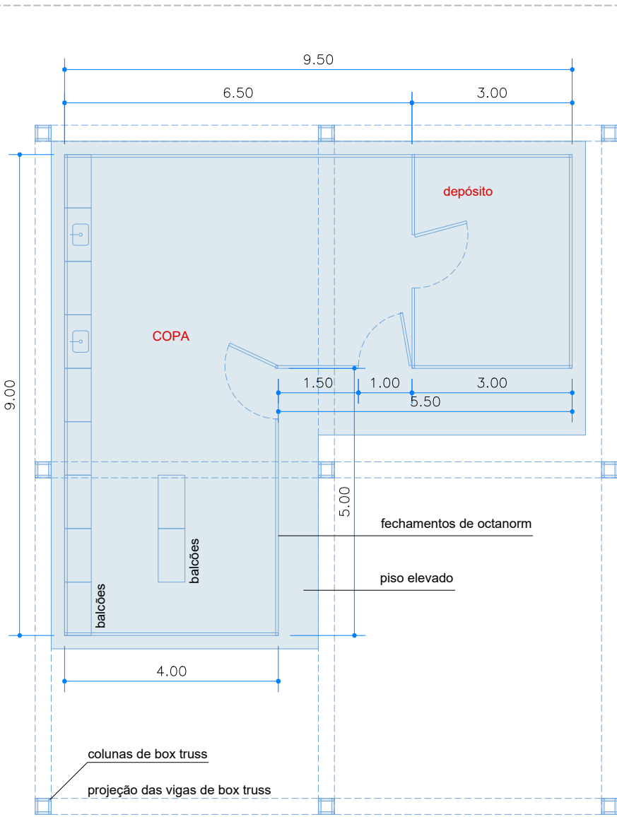
ampliação copa | planta de ambientes de octanorm escala 1:100
