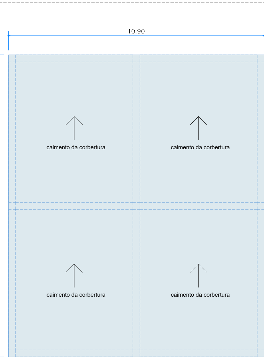
ampliação copa | planta de cobertura com uma água escala 1:100
