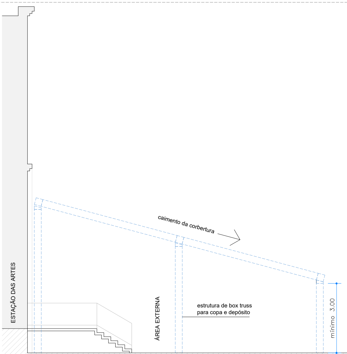
ampliação copa | elevação lateral da tenda de box truss escala 1:100
