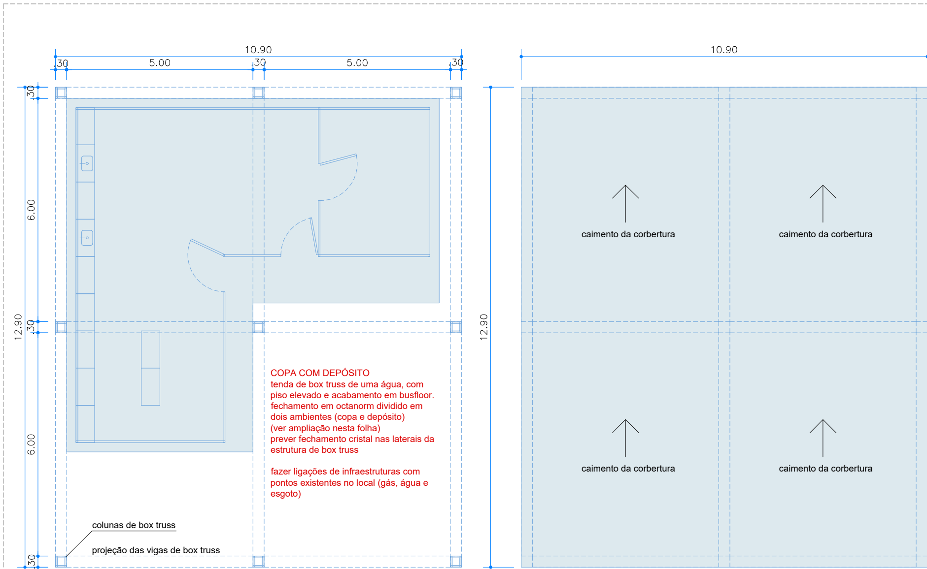
ampliação copa | planta geral escala 1:100
