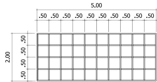
PLANTA ESTRUTURA METALON 40x40mm
