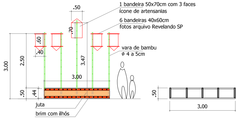
VISTA FRONTAL (fechamento da estrutura)
