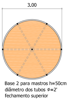
VISTA SUPERIOR (estrutura)
