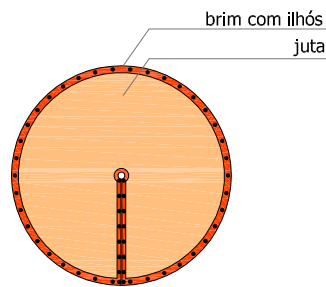
VISTA SUPERIOR (fechamento da estrutura)
