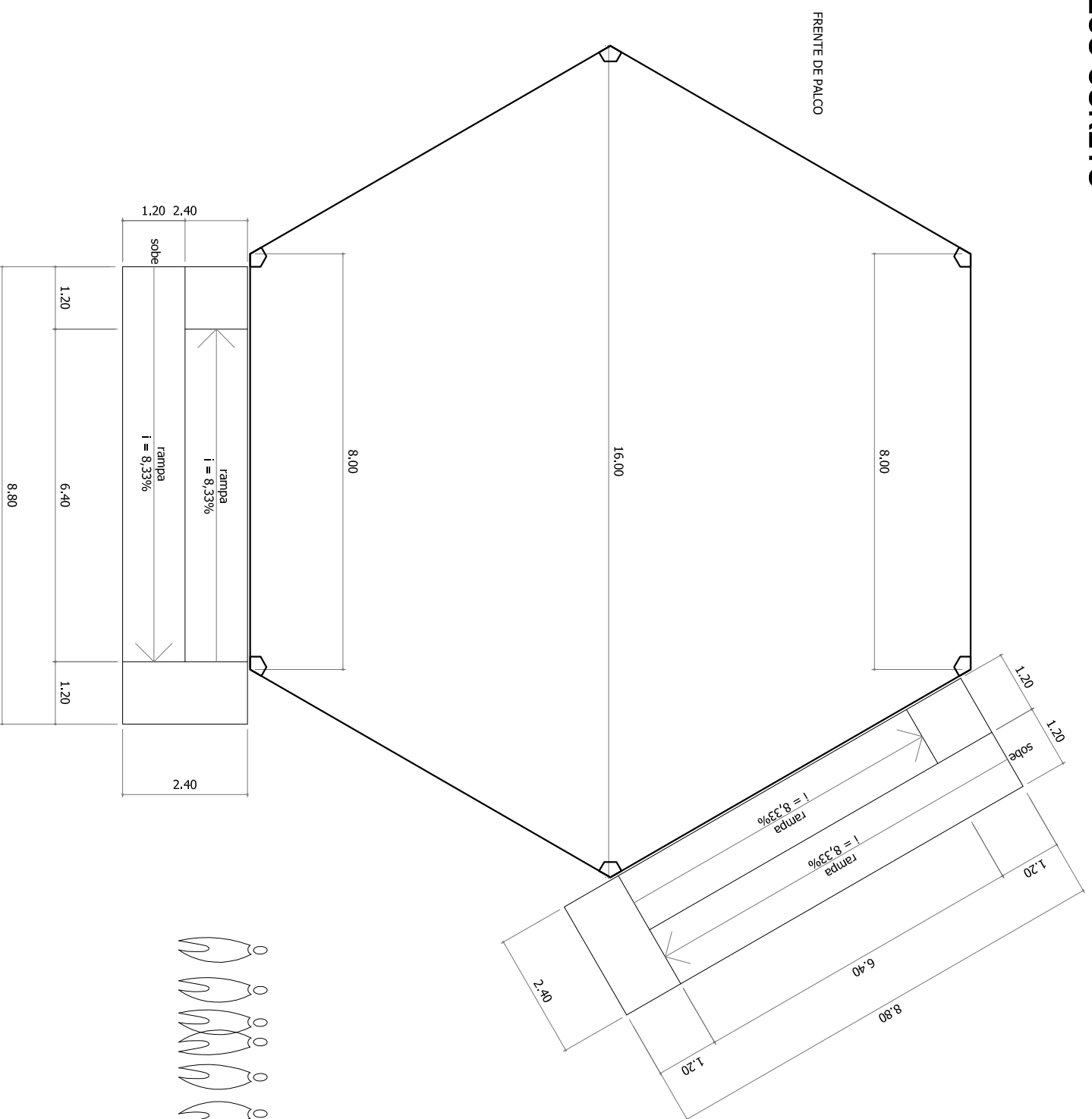
PLANTA ESQUEMÁTICA (com acesso por rampas laterais)
