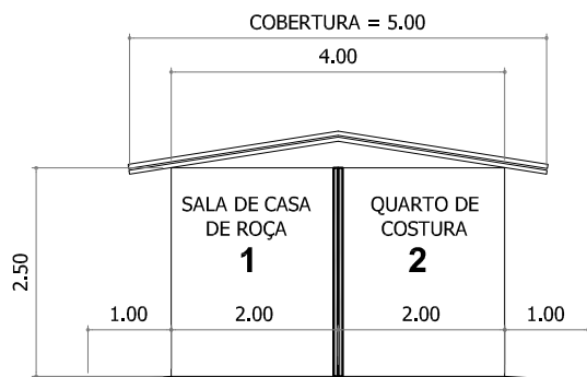
CONJUNTO 1 SALA / QUARTO DE COSTURA CORTE ESQUEMÁTICO
