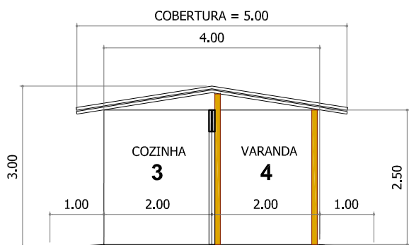
CONJUNTO 2 COZINHA / VARANDA CORTE ESQUEMÁTICO
