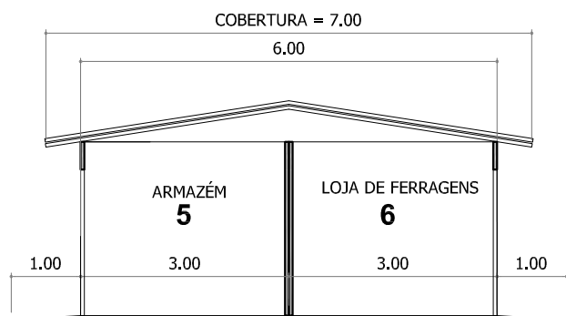
CONJUNTO 3 ARMAZÉM / LOJA DE FERRAGENS CORTE ESQUEMÁTICO
