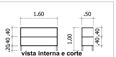
vista interna e corte
