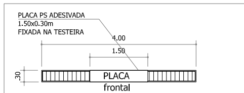
vista testeira frontal COM placa
