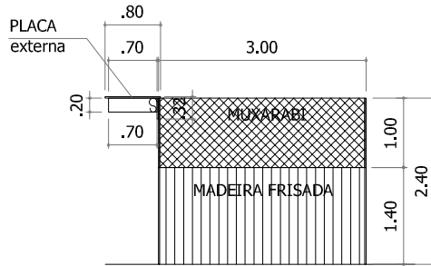
VISTA PAREDE LATERAL
