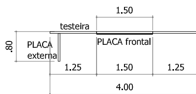
PLANTA TESTEIRA E PLACAS
