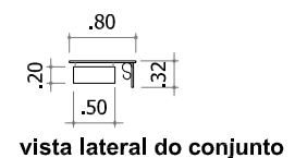
vista lateral do conjunto
