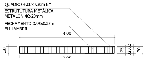
vista testeira frontal
