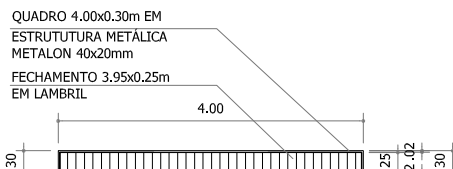
vista testeira frontal
