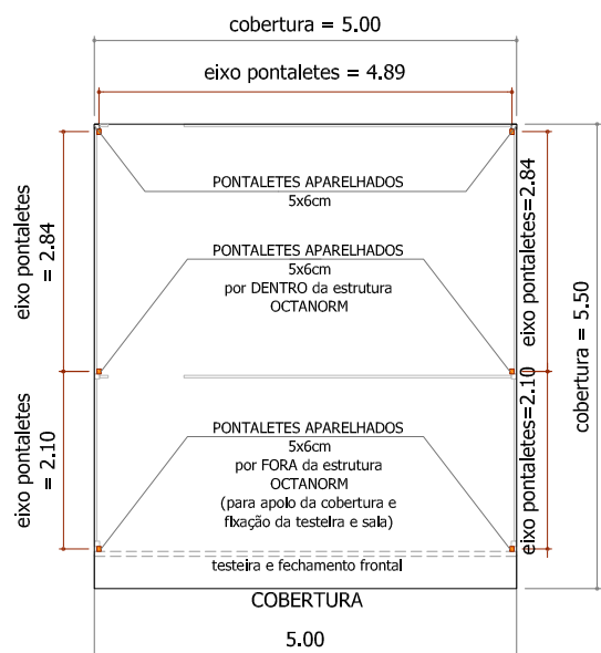
PLANTA ESTRUTURA COBERTURA
