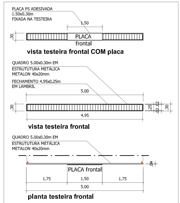
TESTEIRA (detalhamento) cor estrutura metálica: marrom café cor lambril de madeira: amarelo jasmim
