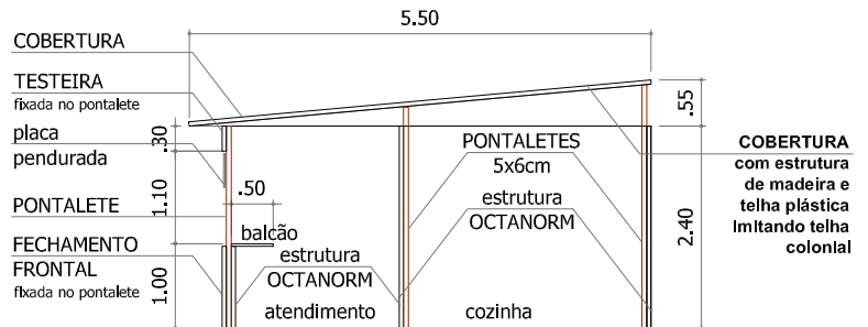
CORTE ESQUEMÁTICO
