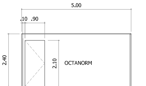
VISTA INTERNA
