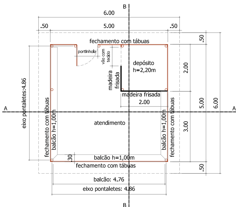
PLANTA
