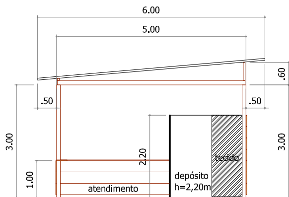
CORTE B-B
