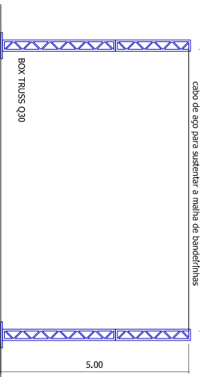
CORTE ESQUEMÁTICO
