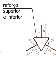
PLANTA ESTRUTURA BARRA CHATA (22x10mm)
