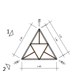
PLANTA COMPLETA TRÍPTICO (3 faces de 1.49m)
