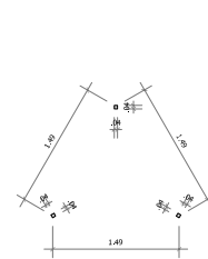
PLANTA COLUNAS VERTICAIS METALON (40x40mm)
