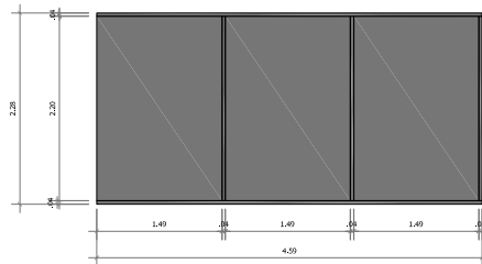
VISTA TECIDO PARA 3 IMAGENS (abraçando a estrutura) dimensão total: 4.59 x 2.28m
