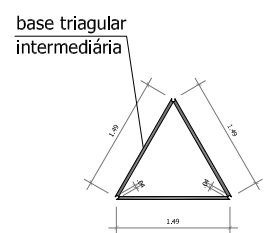
PLANTA REFORÇO INTERMEDIÁRIO METALON (40x40mm)
