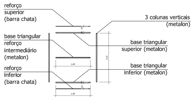
CORTE ESTOURADO
