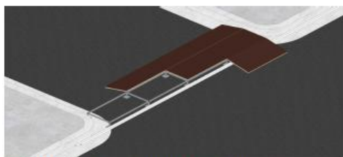
AMPLIAÇÃO DA RAMPA - VISUALIZAÇÃO DOS ELEMENTOS piso elevado modular com pés metálicos reguláveis, chapeamento de madeira e revestimento de piso easyfloor de rolo, com acabamento rampado
