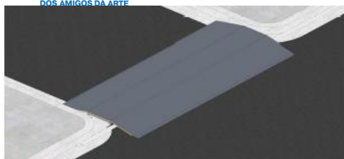
AMPLIAÇÃO DA RAMPA piso elevado modular com pés metálicos reguláveis, chapeamento de madeira e revestimento de piso easyfloor de rolo, com acabamento rampado
