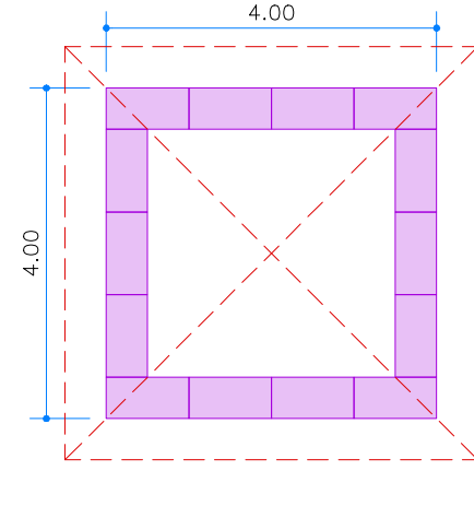
BALCÕES PARA BAR 4x4m PLANTA ESCALA 1:100 05 unidades
