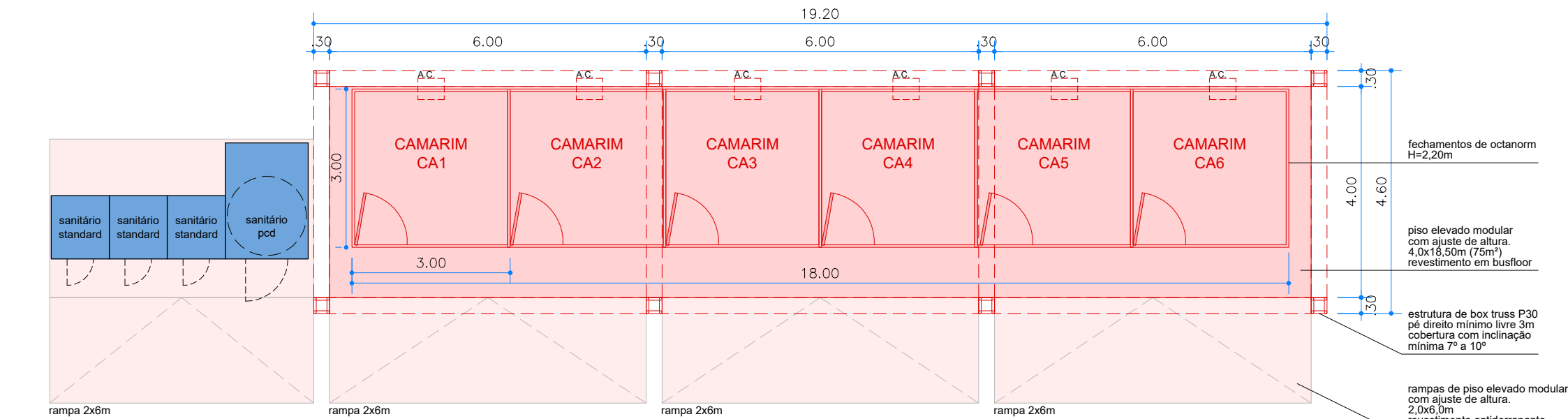
CAMARINS 1 PLANTA ESCALA 1:100 FECHAMENTOS EM OCTANORM, H=2,20m (PREVER COBERTURA E AR-CONDICIONADO) (INSTALADO SOBRE PISO ELEVADO MODULAR EM ESTRUTURA DE BOX TRUSS P30)
