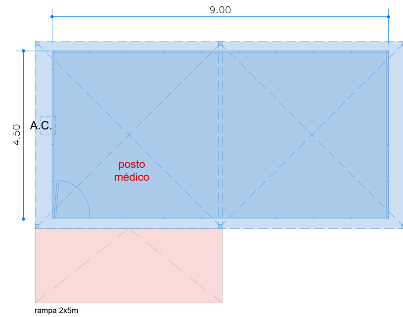
POSTO MÉDICO ESCALA 1:100 FECHAMENTOS EM OCTANORM, H=2,20m INSTALAÇÃO SOBRE PISO MODULAR COM REVESTIMENTO EM BUSFLOOR (VERIFICAR MEDIDAS NO LOCAL E ADAPTAR FORMATO, CASO NECESSÁRIO) (PREVER COBERTURA E AR-CONDICIONADO)
