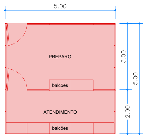
ESTANDE ALIMENTAÇÃO COM PREPARO 5x5m ESCALA 1:100 10 UNIDADES
