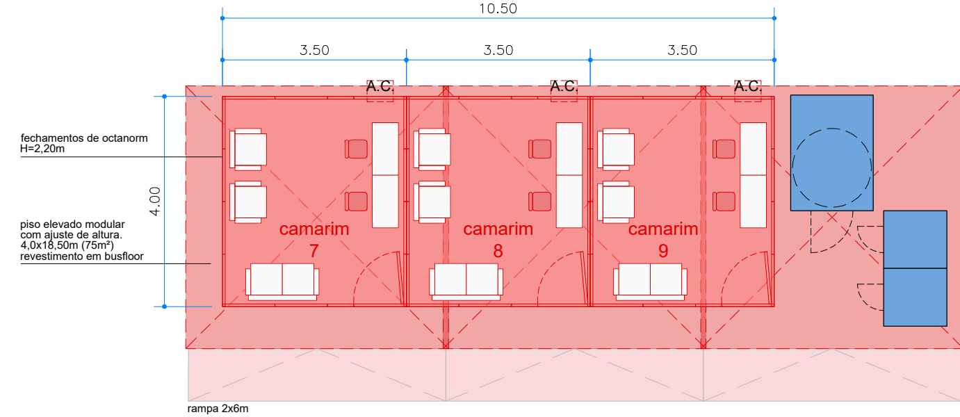
CAMARINS 2 PLANTA ESCALA 1:100 FECHAMENTOS EM OCTANORM, ALTURA=2,20m (PREVER COBERTURA E AR-CONDICIONADO) (INSTALAÇÃO SOBRE PISO ELEVADO MODULAR E SOB TENDAS 5x5m)
