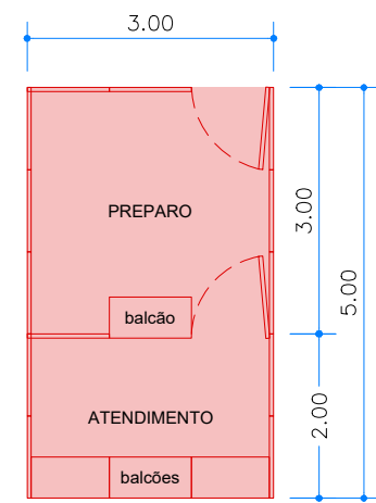
ESTANDE ALIMENTAÇÃO COM PREPARO 3x5m ESCALA 1:100 14 UNIDADES
